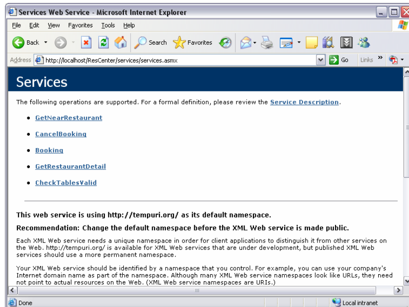
รูป 4.15 ภาพแสดงตัวอย่างเซอร์วิสของเว็บเซอร์วิสร้านอาหารที่เปิดให้เว็บเซอร์วิส Smart Tour Agency เรียกใช้
