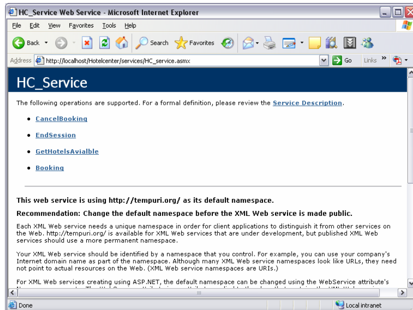
รูป 4.13 ภาพแสดงตัวอย่างเซอร์วิสของเว็บเซอร์วิสโรงแรมที่เปิดให้เว็บเซอร์วิส Smart Tour Agency เรียกใช้
